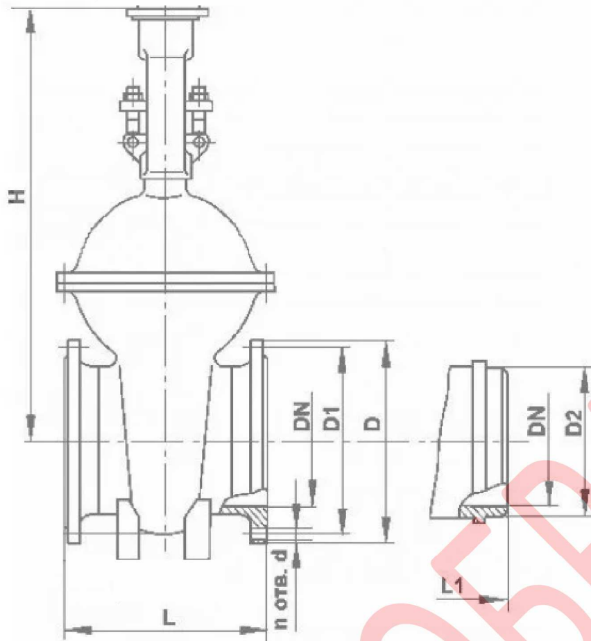
Габаритные и присоединительные размеры, масса
