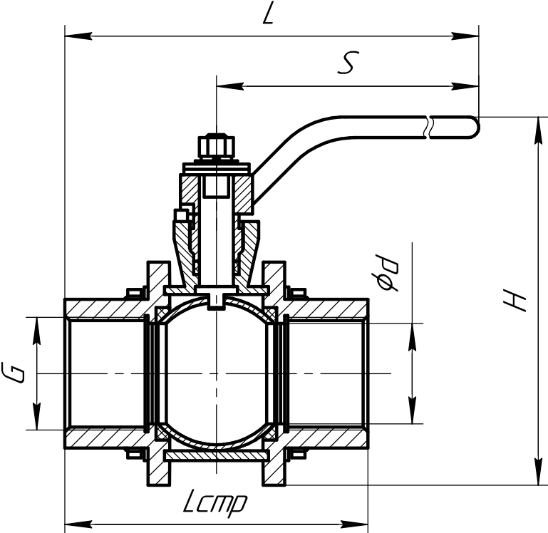
Трёхсоставная конструкция корпуса Краны шаровые Ду свыше 40 мм
