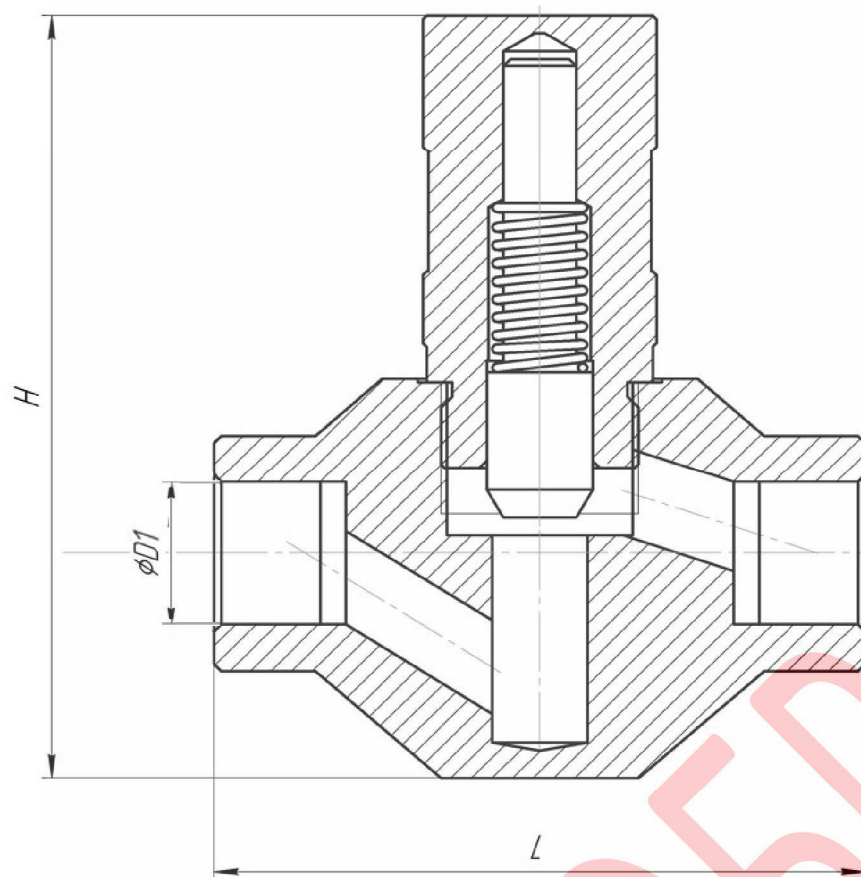
Габаритные и присоединительные размеры, масса
