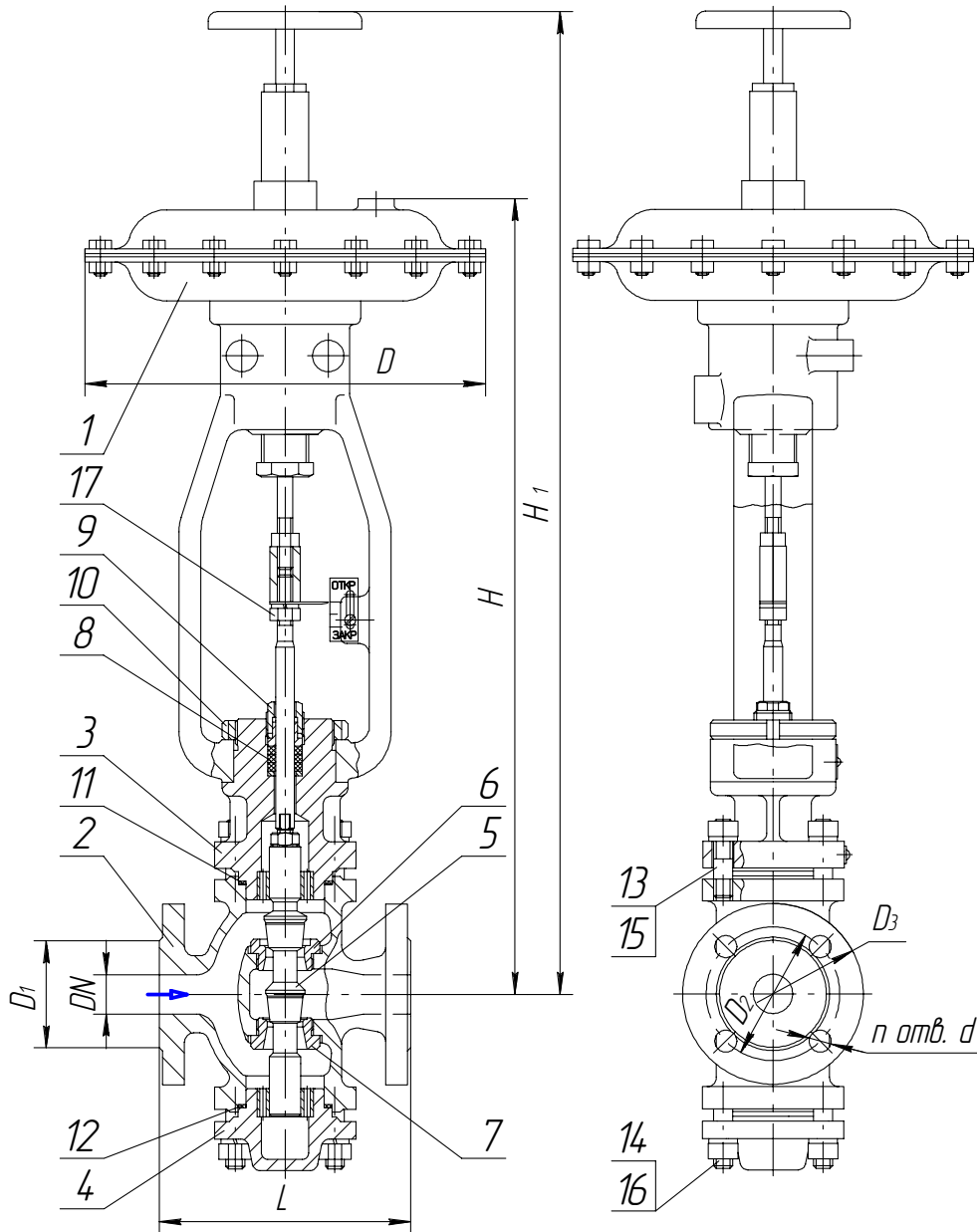
Рисунок 1 Основные узлы и габариты клапана HO
