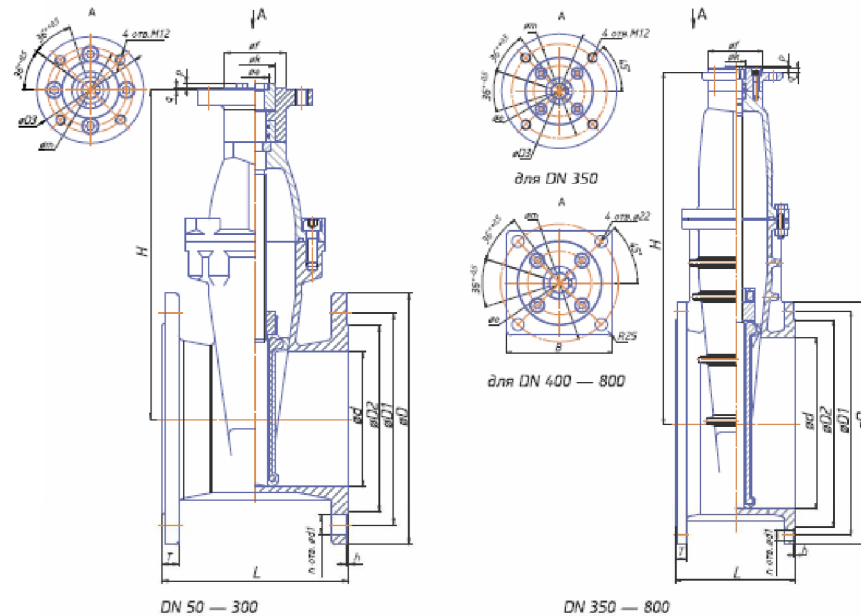
Габаритные и присоединительные размеры, масса
