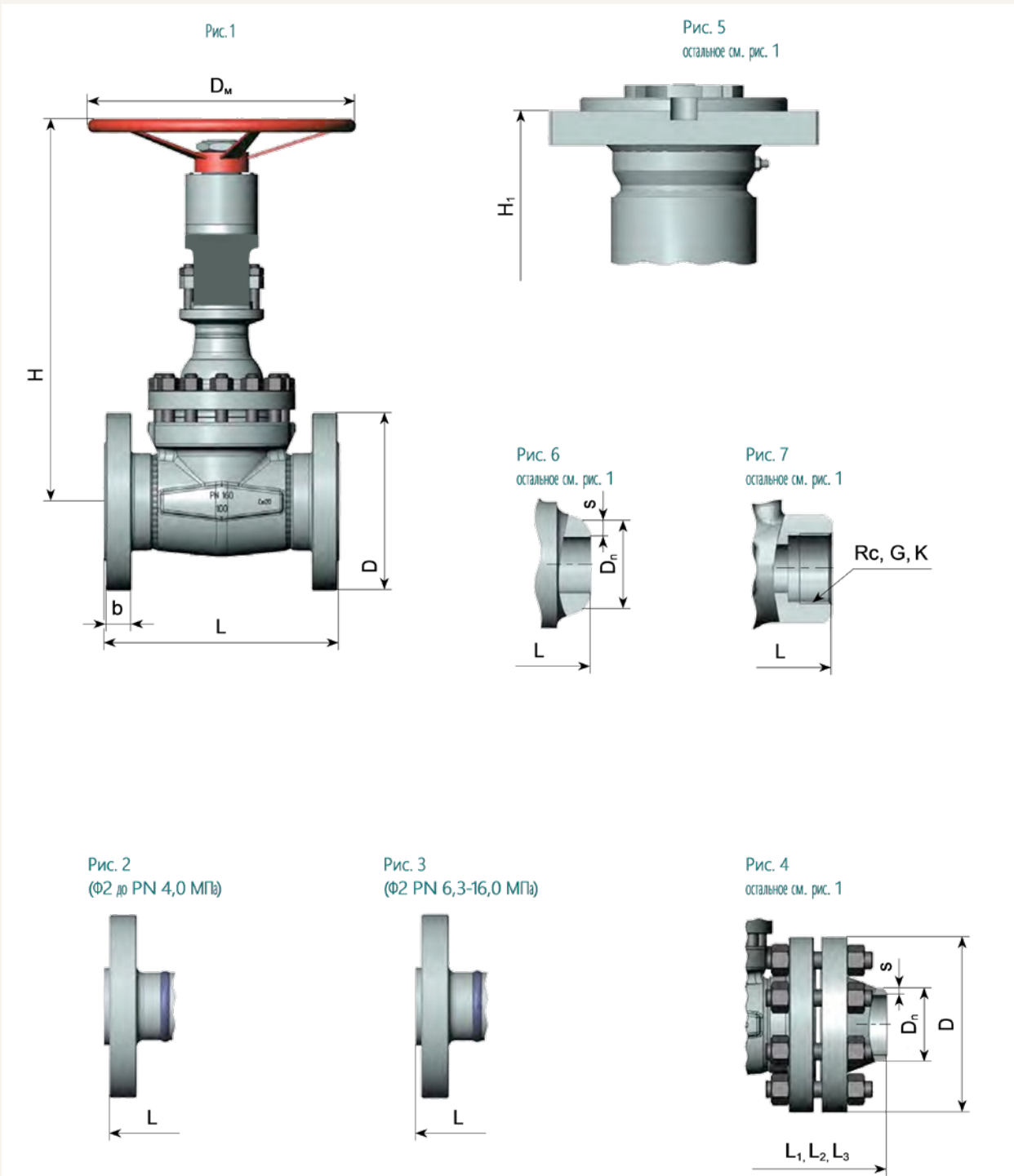
ОСНОВНЫЕ РАЗМЕРЫ, ММ Задвижки присоединения под приварку встык
