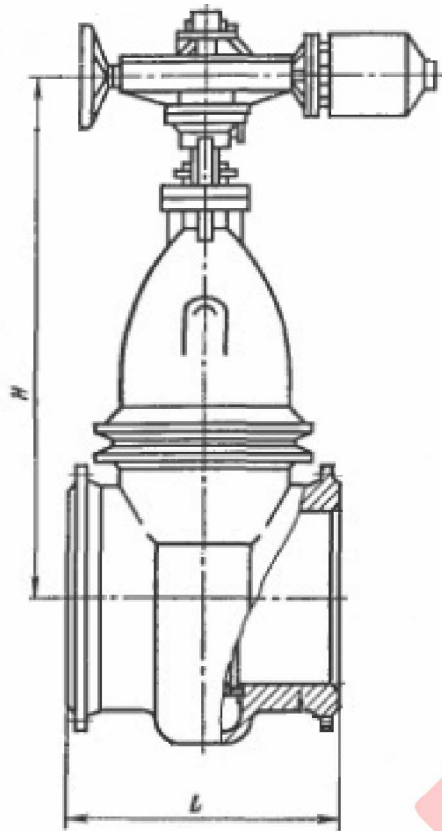
Габаритные размеры, масса
