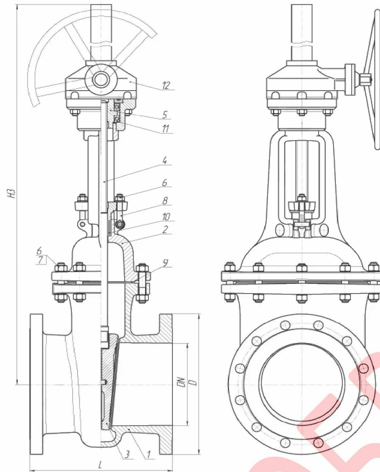
Габаритные и присоединительные размеры, масса
